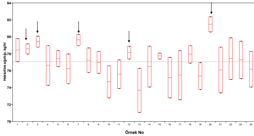
Şekil 3. Kuru ve suluda örneklere ait hektolitre ağırlığı değerlerinin değişimi
