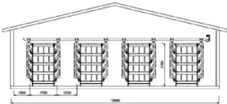
Şekil 2. Katlı Kafes Sistemi
